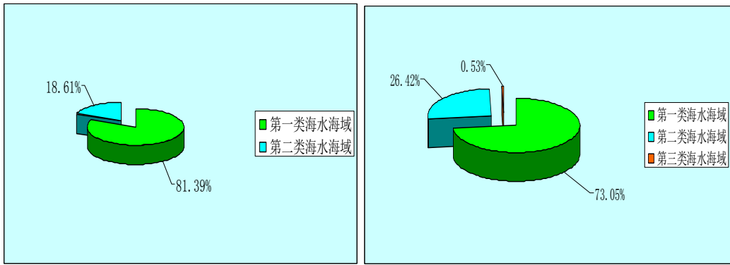
2014年春季重点港湾水质状况分布图 2014年夏季重点港湾水质状况分布图
