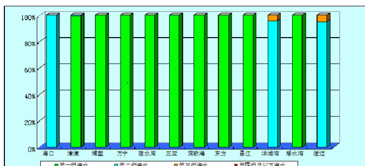
2014年夏季各重点港湾海水水质状况对比图
