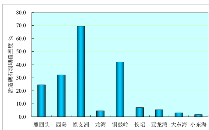
2014年海南省东海岸造礁石珊瑚覆盖度
